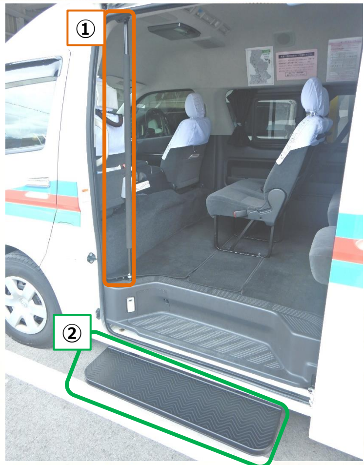
滋賀県米原市の「まいちゃんバス」乗 降口に取り付けた1段のグリップ（握 り棒）と昇降ステップ
